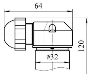
Рисунок 2 С угловым пластмассовым (УП) сальниковым вводом остальное см.рис1
