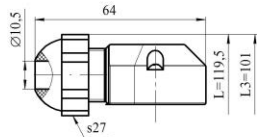
Рисунок Г18 остальное см. рисунки Г14-Г17
