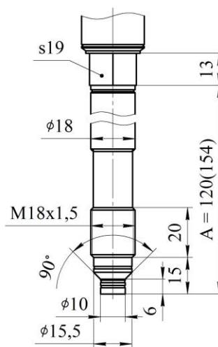
Рисунок 6 Резьба М18х1,5 остальное см.рис1
