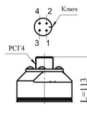
Рисунок Г13 остальное см. рисунки Д9-Д11
