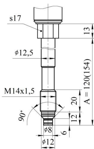
Рисунок 5 Резьба М14х1,5 остальное см.рис1
