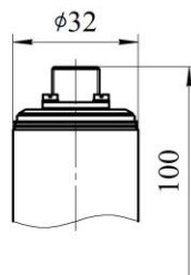
Рисунок 3 С разъемом РСГ7ТВ (Р) остальное см.рис1
