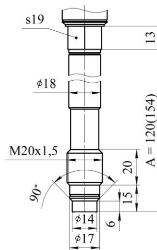
Рисунок 7 Резьба М20х1,5 остальное см.рис1
