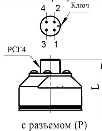
Рисунок Г4 Остальное см. рисунки Г1, Г2
