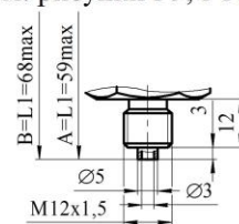
Рисунок Г12 остальное см. рисунки Г9-Г11
