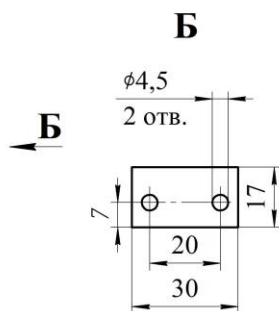
Рисунок 5 Резьба М14х1,5 остальное см.рис1
