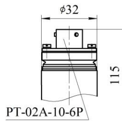
Рисунок 4 С разъемом РТ-02А-10-6Р (Р6) остальное см.рис1
