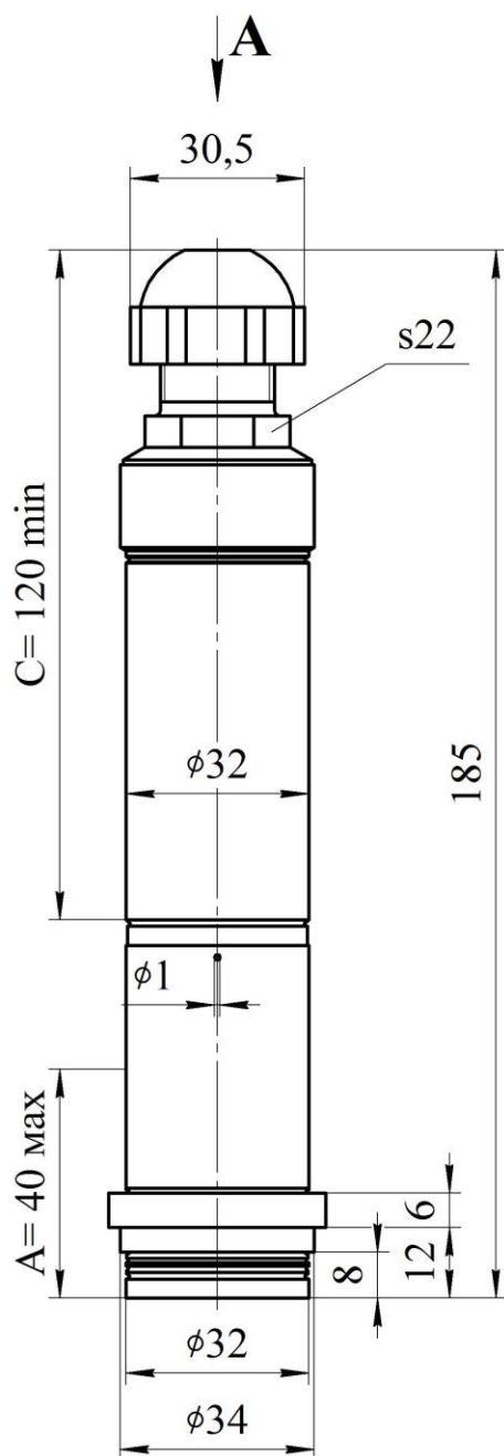
Рисунок 1 С прямым металлическим (ПМ) сальниковым вводом
